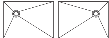
PCI Pecibord® Rechteck, Ablauf decentral oben links/rechts Brodzik prostokątny. Odpływ: usytuowany decentralnie
